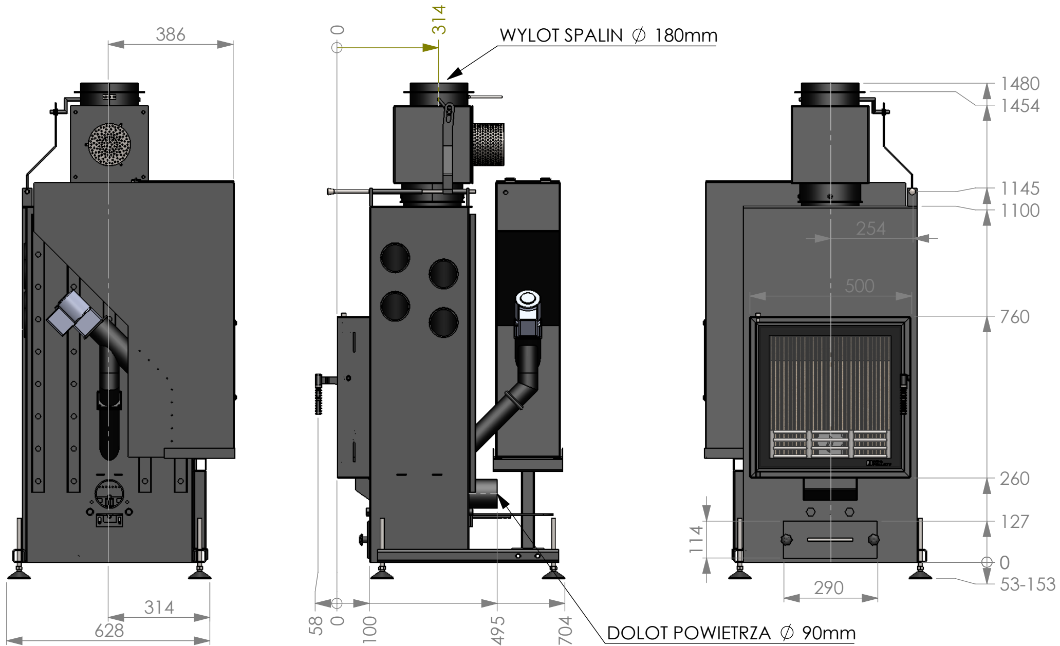
WYMIARY - ALEX AIR 10kW
